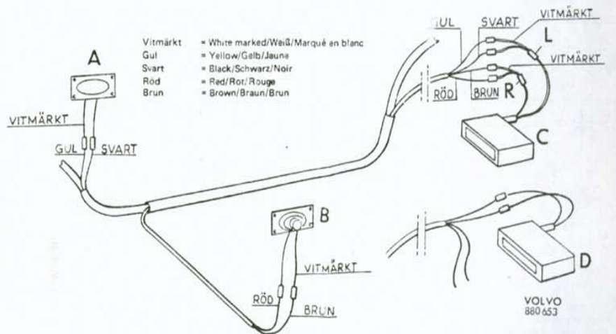
Fig. 5 Kopplingschema
