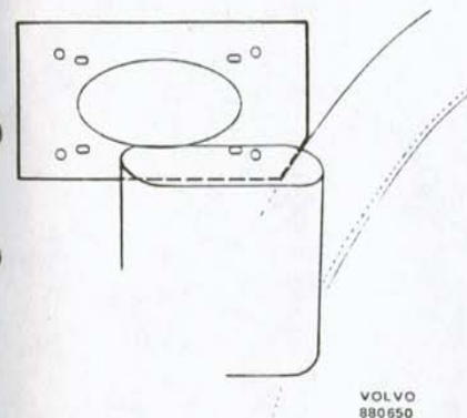
Fig. 2 Placering av mall Fig. 2 Placing the template Abb. 2 Anbringning der Vorlage Figure 2 Emplacement du gabarit de perçement
