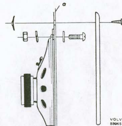
Fig. 3 Fastsättning av högtalare och högtalargaller a = sidopanel Fig. 3 Fixing on the speaker and speaker grille a = side panel Abb. 3 Befestigung von Lautsprecher und Lautsprechergitter a = Seitenverkleidung Figure 3 Fixation du haut-parleur et de la grille de haut-parleur a = Panneau latéral
